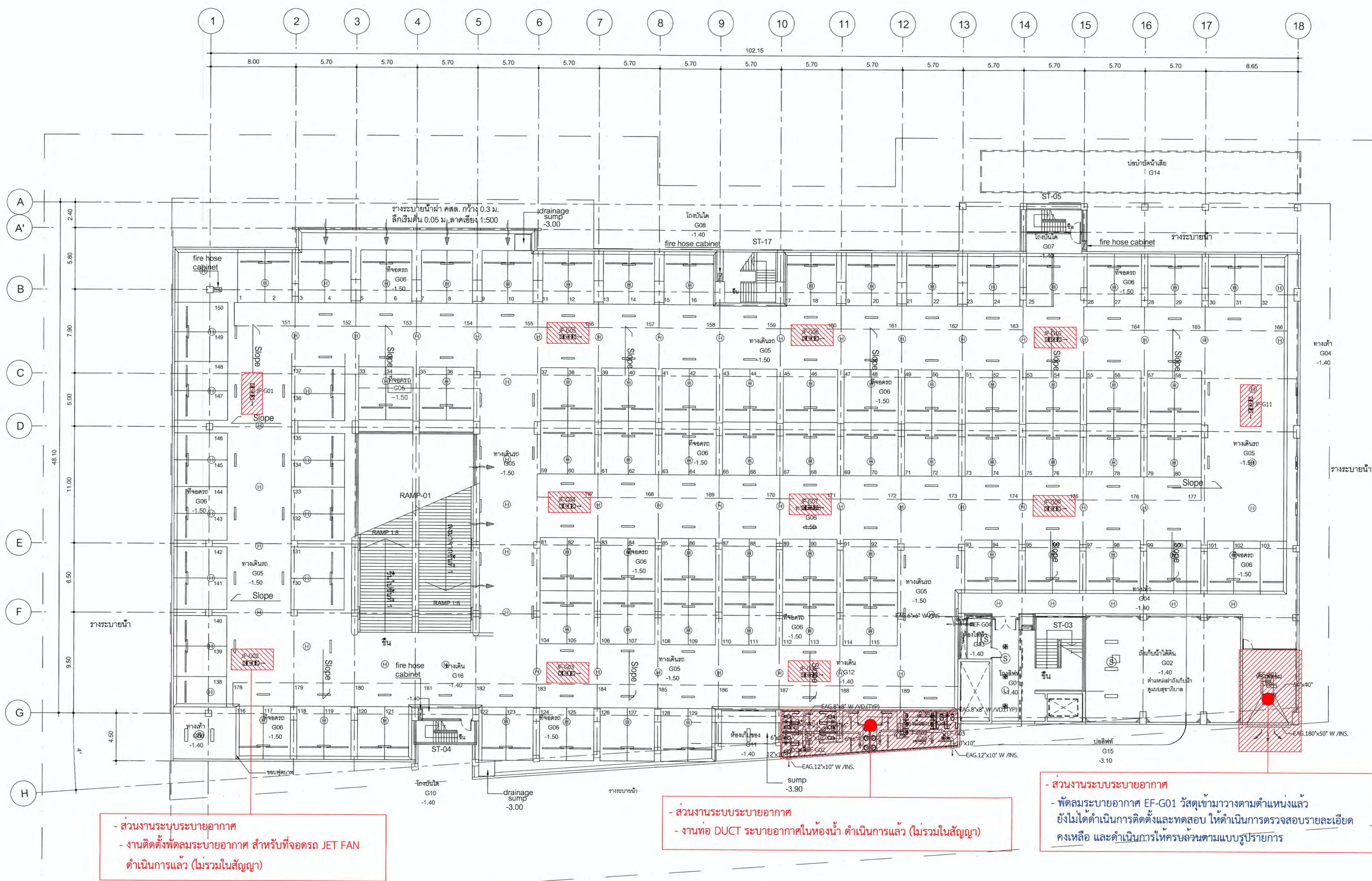
ผังงานท่อลมระบบปรับอากาศและระบายอากาศชั้นล่าง SCALE 1 : 200
