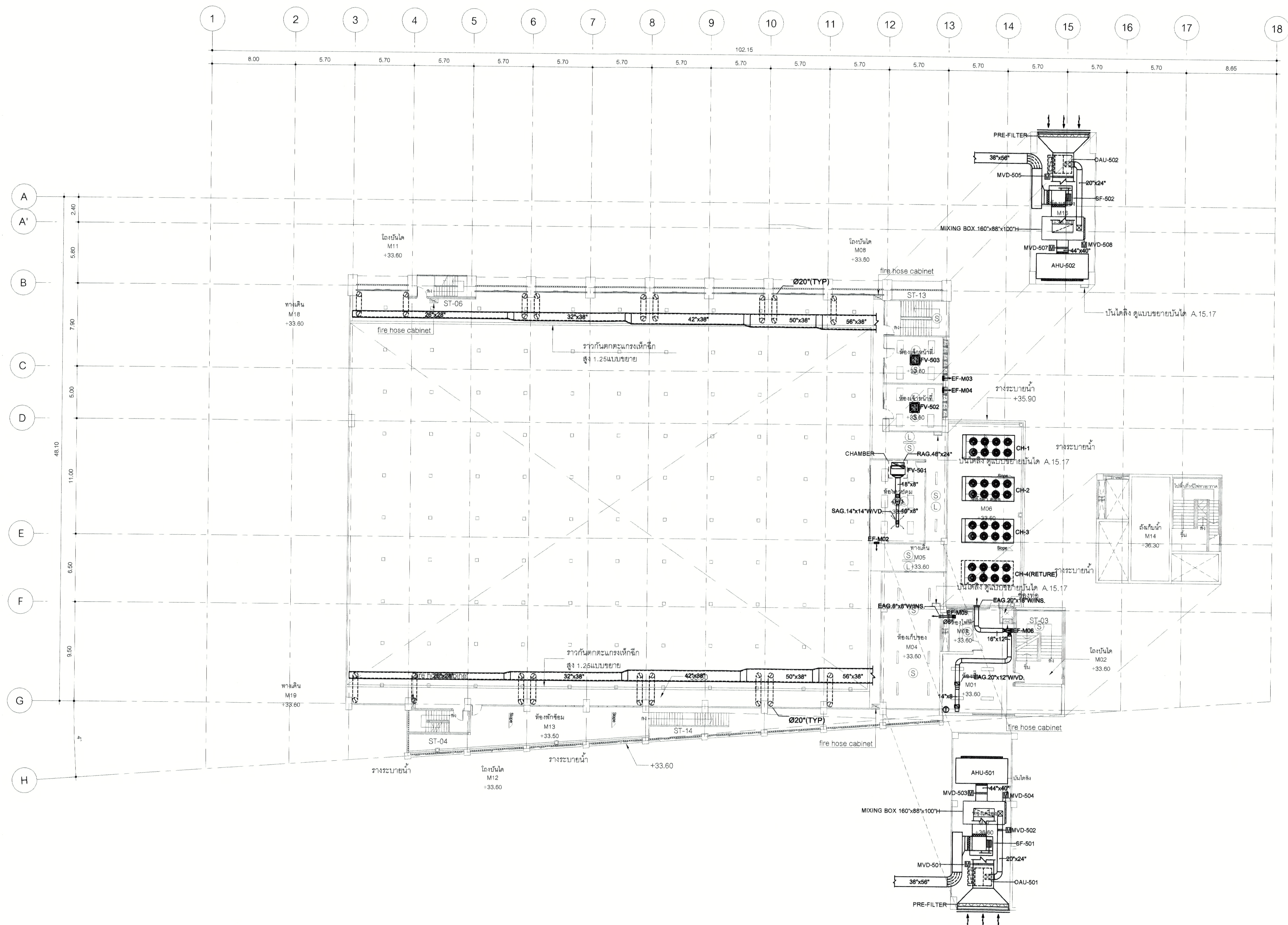
ผังงานท่อลมระบบปรับอากาศและระบายอากาศชั้นที่ MEZZANINE SCALE 1 : 200
